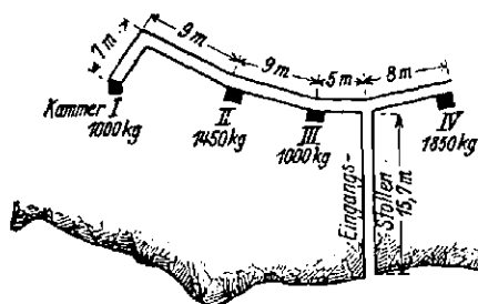
Lageplan 1:250
