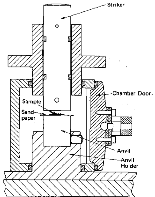
Fig 1. Anvil Striker Arrangement, ERL Machine
