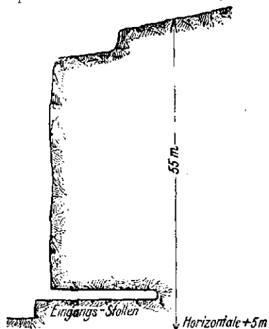
Schnitt durch den Eingangsstollen 1:250
