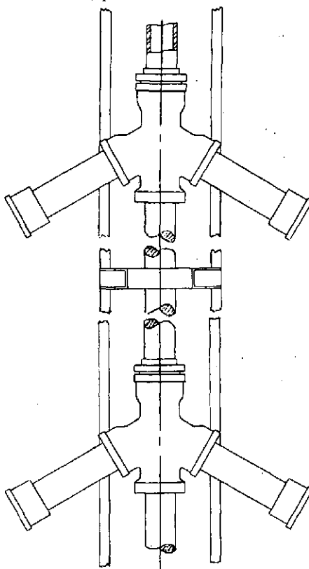
HDP Supergun (Vergeltungswaffe 3) (V-3)
